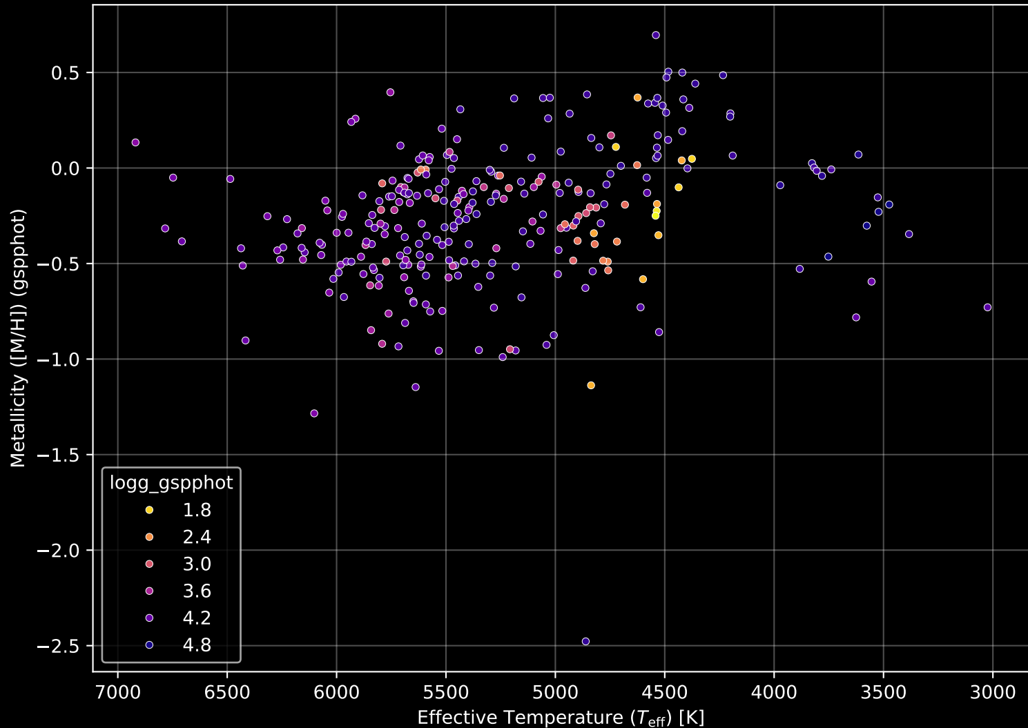
APOGEE DR17 Field: [sgr_tidal4] Stellar Population Parameters (n= 288)
